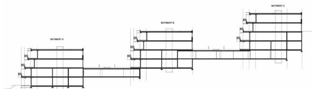
Coupe transversale
